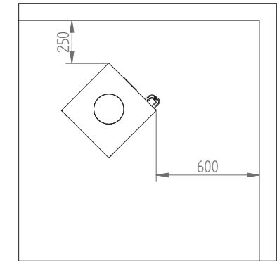
Panorama avstånd till brännbart utan isolerad skorsten
