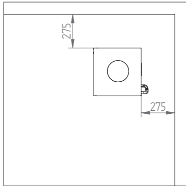
Panorama avstånd till brännbart med isolerad skorsten
