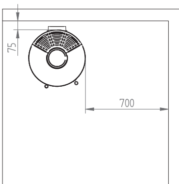
EOS avstånd till brännbart med isolerad skorsten
