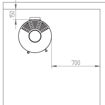
EOS avstånd till brännbart utan isolerad skorsten
