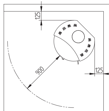
Cubic avstånd till brännbart utan isolerad skorsten
