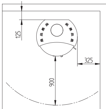
Cubic avstånd till brännbart med isolerad skorsten
