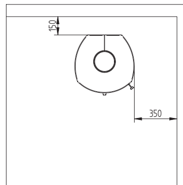
Senza avstånd till brännbart med/utan isolerad skorsten
