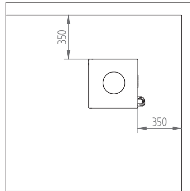
Panorama avstånd till brännbart utan isolerad skorsten
