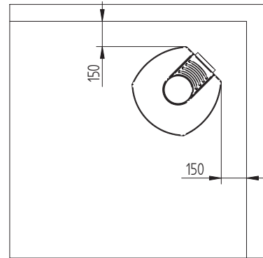
Country 575/765 avstånd till brännbart med/utan isolerad skorsten
