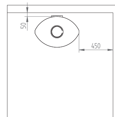
Elegance avstånd till brännbart med isolerad skorsten
