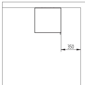
Mido avstånd till brännbart utan isolerad skorsten
