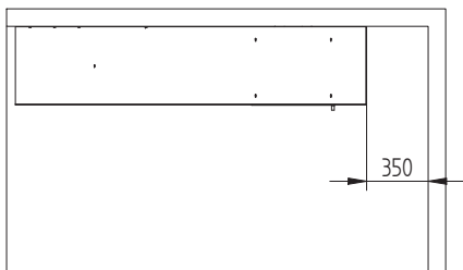
Cubic W200 avstånd till brännbart med/utan isolerad skorsten
