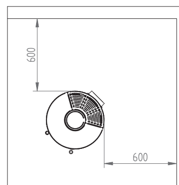
EOS avstånd till brännbart med/utan isolerad skorsten
