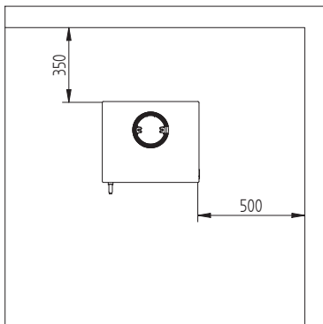
Country 575/765 avstånd till brännbart utan isolerad skorsten
