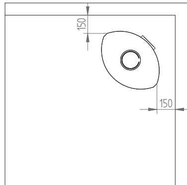
Cosmo avstånd till brännbart med isolerad skorsten
